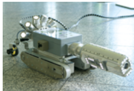
Bild 1: Der Inspektions-Prototyp findet mit hochauflösenden Kameras selbst kleine Schadstellen in den Rotorblättern von Windkraftanlagen.
